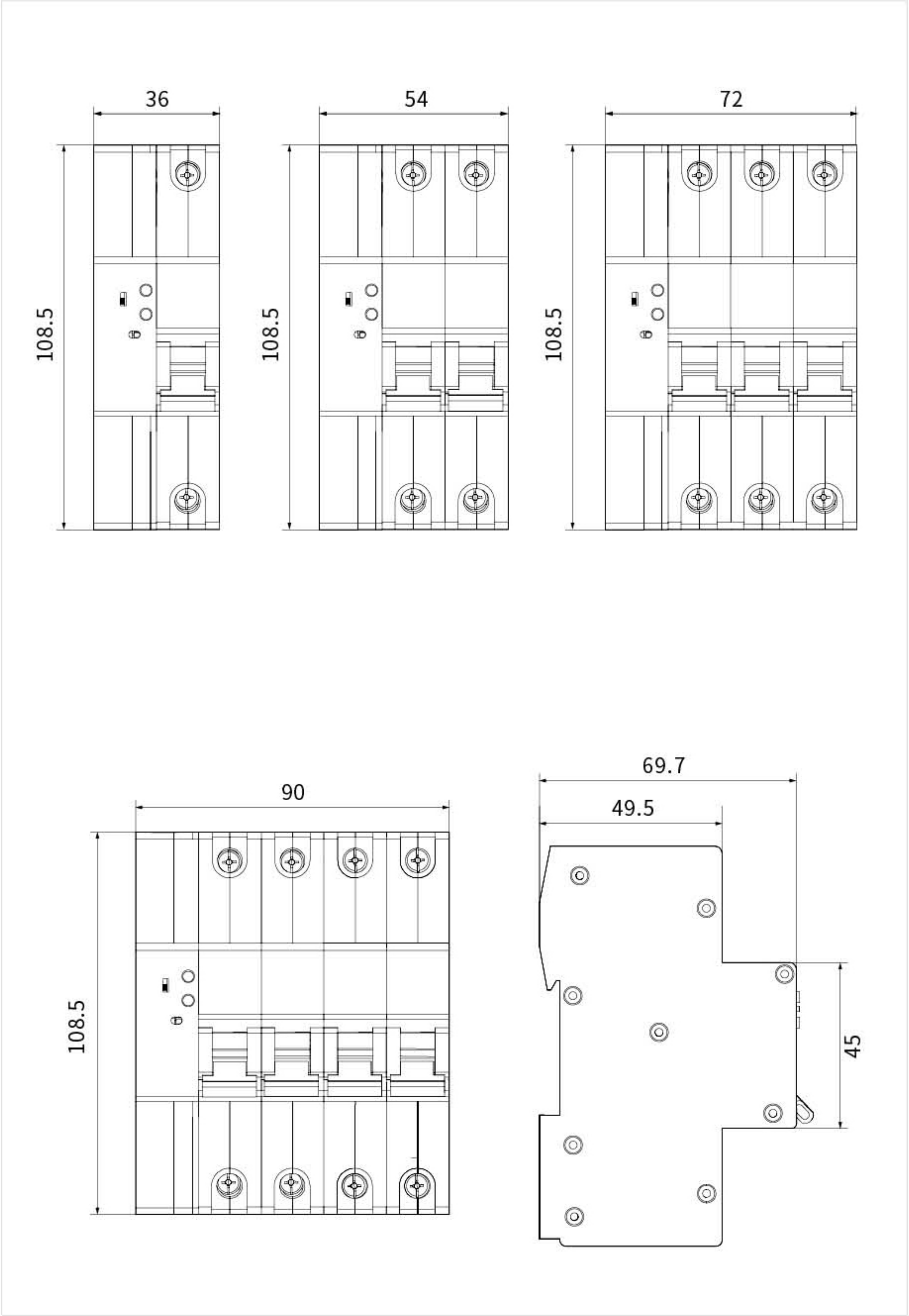
外形及安装尺寸 ( mm )
